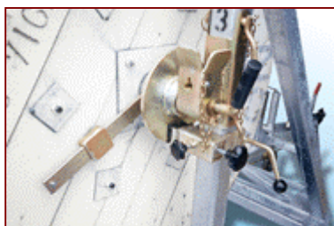
Frein à disque Scheibenbremse REF. 18-9920
